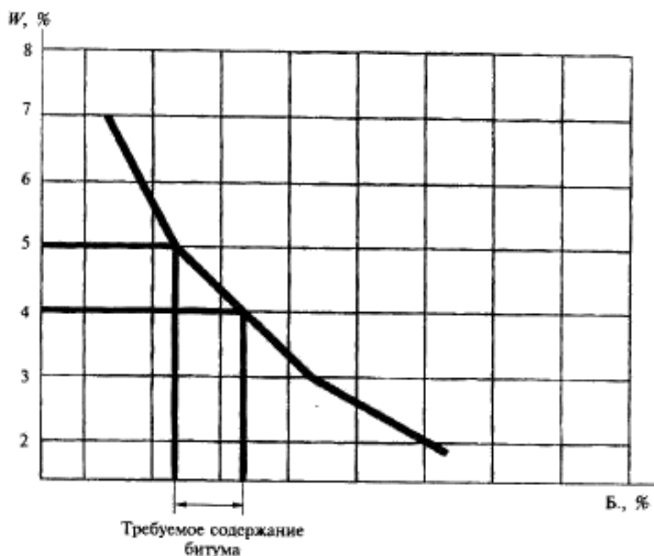
Рисунок 3 — Определение требуемого содержания битума
